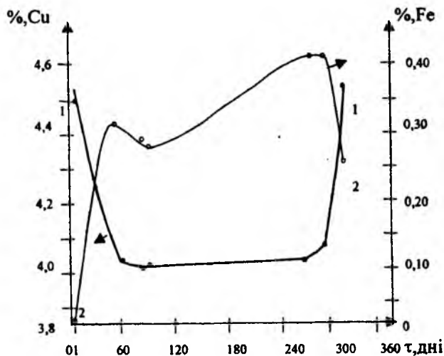
Рис.1. Залежність вмісту основних компонентів промислової партії каталізатора оксихлорування етилену від терміну роботи реактора:
