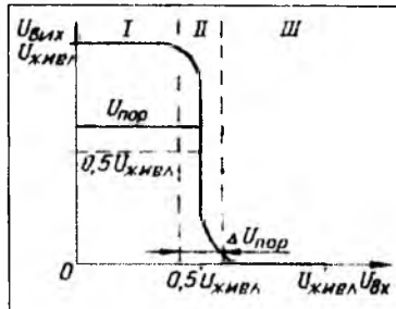
Рис. 1. Передаточна характеристика одиночного інвертора.
